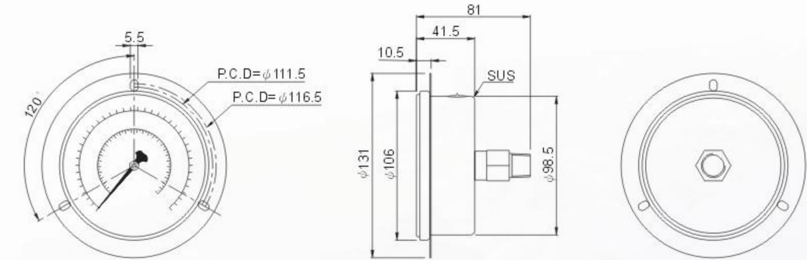
AE-AF/4 . AE-AFK/4 . BE-AF/4
