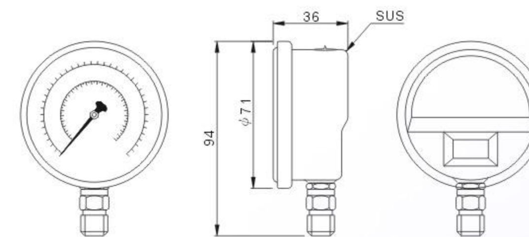
AC-A/25 . AC-AK/25 . BC-A/25
