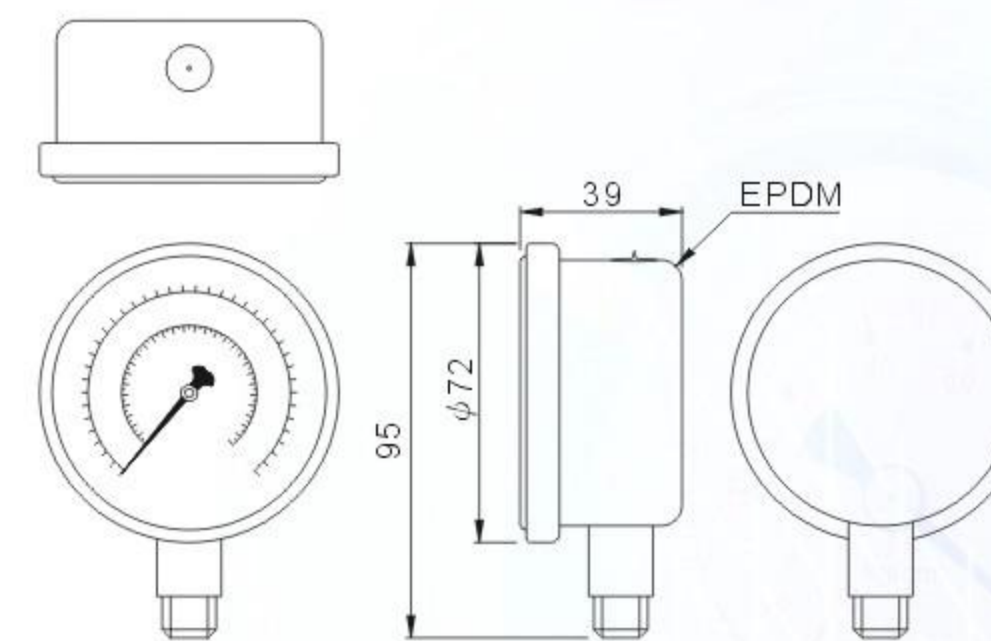
AC-AB/25 . AC-ABK/25 . BC-AB/25
