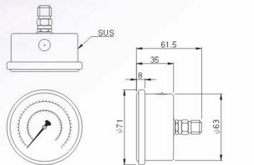
AE-A/25 . AE-AK/25 . BE-A/25
