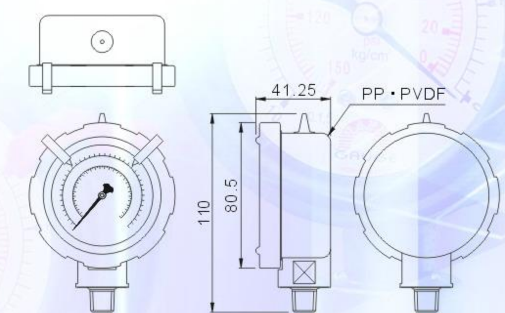
AD-A/25 . AD-AK/25 . BD-A/25
