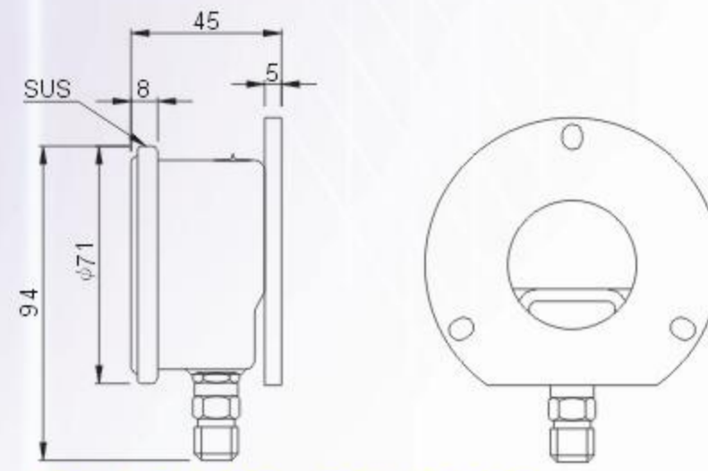
AC-AF/25 . AC-AFK/25 . BC-AF/25
