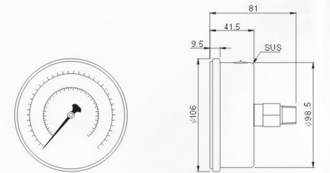
AE-AK/4 . AE-A/4 . BE-A/4
