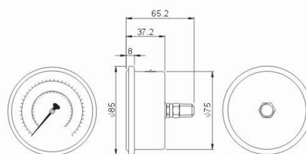
AE-A/3 . AE-AK/3 . BE-A/3
